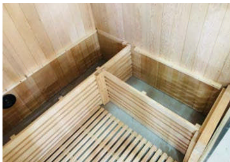
Instalovaná podpora zadního a pravého sedáku
