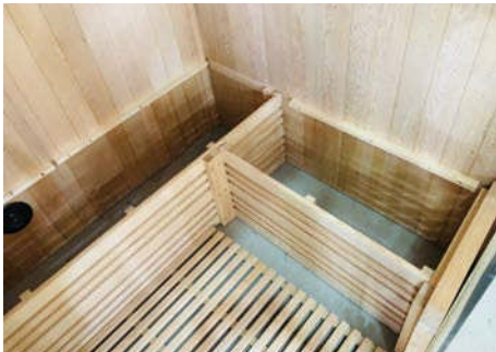
Inštalovaná podpora zadného a pravého sedadla
